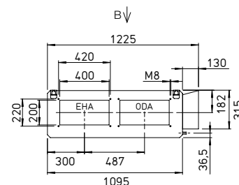
Ansicht D
