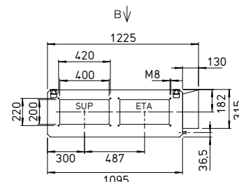
Ansicht D
