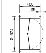
Rohr-Verschlußklappe RVS 630 Nr. 02600
