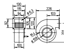
Radial-Kühlluftgebläse B KLG 500 Nr. 02798
