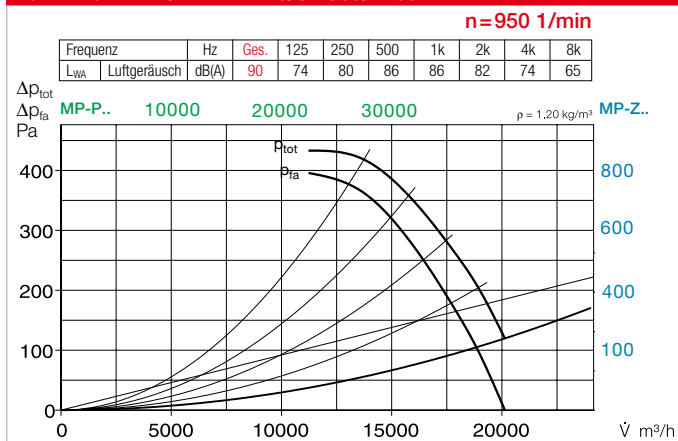
Kennlinien VAR / B VAR 710/6 F300/F400
