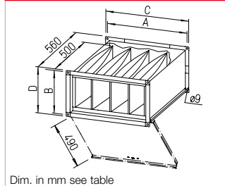
Dimensions KLF F7 2) 3)
