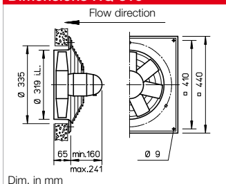
Dimensions HQ 315
