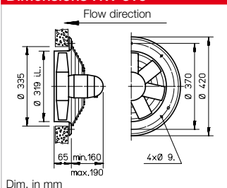
Dimensions HW 315
