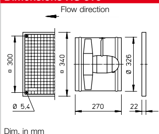
Dimensions HS 315
