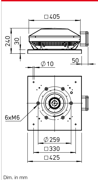
Dimensions RD EC 225
