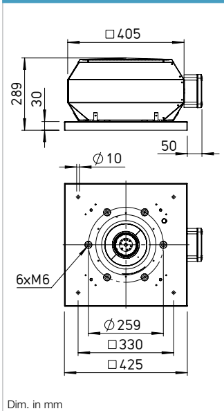
Dimensions VD EC 225
