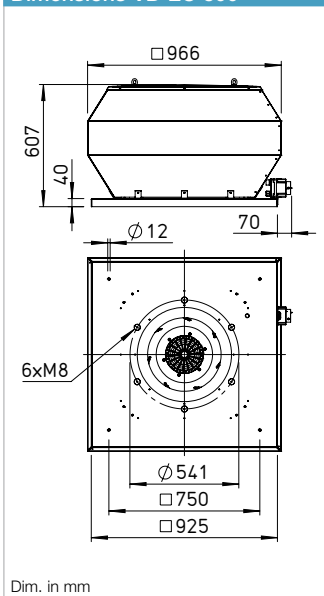
Dimensions VD EC 500
