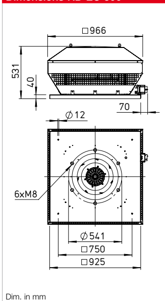
Dimensions RD EC 500
