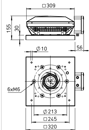
Dimensions RD 180
