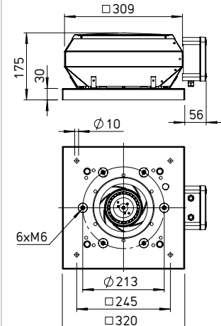
Dimensions VD 180
