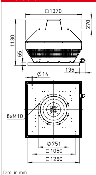
Dimensions RD 710
