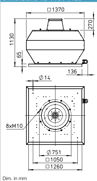
Dimensions VD 710 / T120
