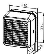
Dimensions GX EC 150
