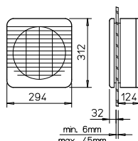
Dimensions GX 225
