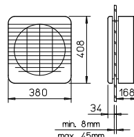
Dimensions GX 300
