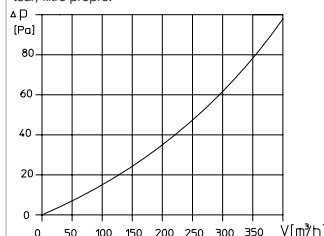
Pertes de charge borne de prise d'air ext. avec filtre ISO Coarse 60 % (G4) et 40 m de collecteur, filtre propre.
