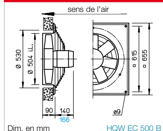
Dimensions HQ EC 500
