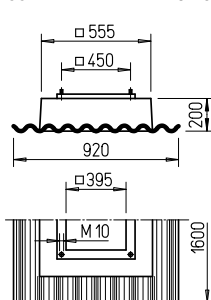
Costière avec silencieux intégré, rabattable SSD 250
