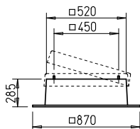
Costière pour toits plats, rabattable FDS 250
