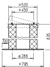
Costière avec silencieux intégré, rabattable SSD 250
