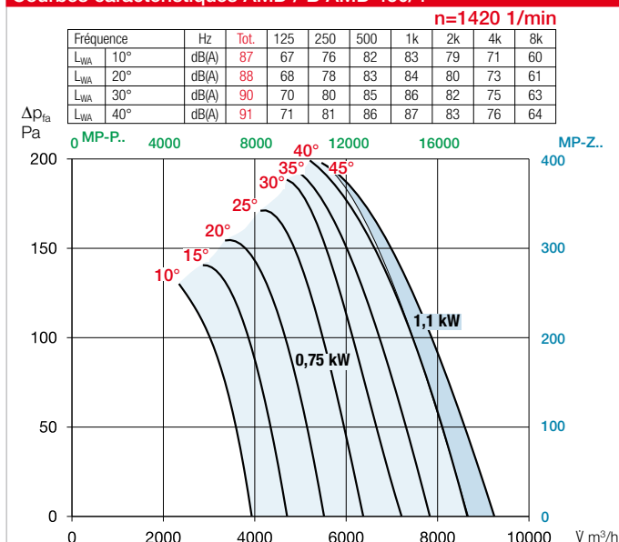
Courbes caractéristiques AMD / B AMD 450/4
