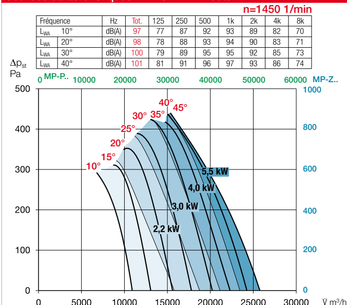
Courbes caractéristiques AMD / B AMD 630/4
