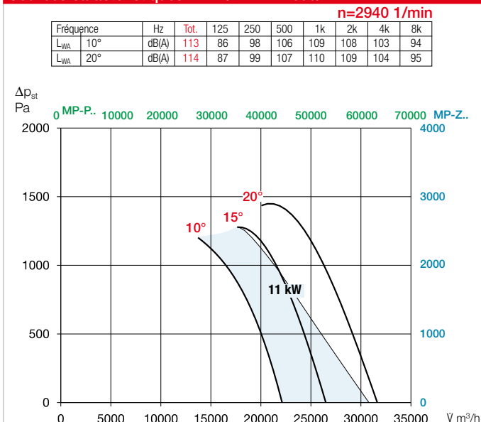
Courbes caractéristiques AMD / B AMD 630/2
