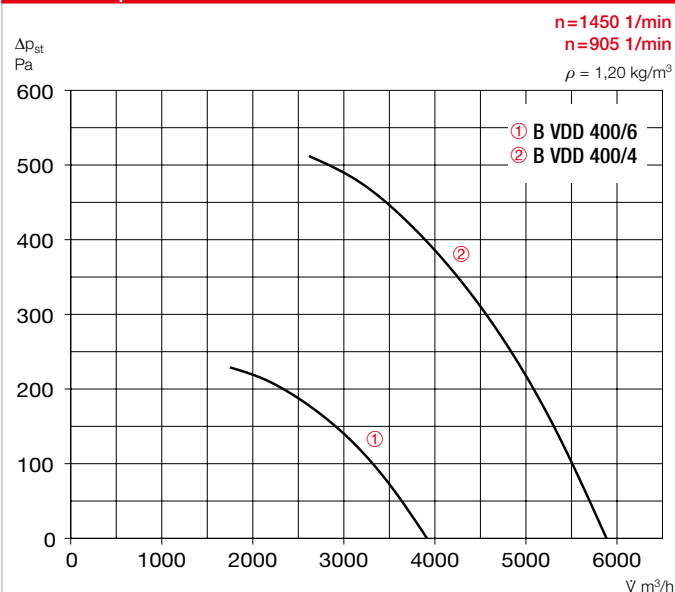
Courbe de performances B VD 400 F400/F600
