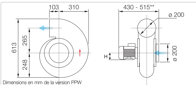
Dimensions en mm de la version PPW
