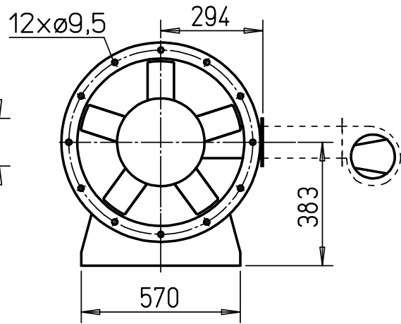
Zubehör MK 500-560
