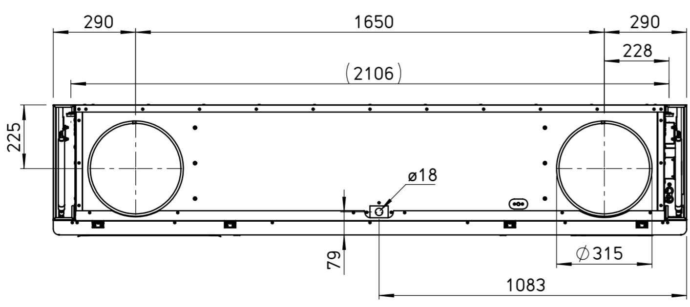
Ansicht mit Kondensatanschluss unten
