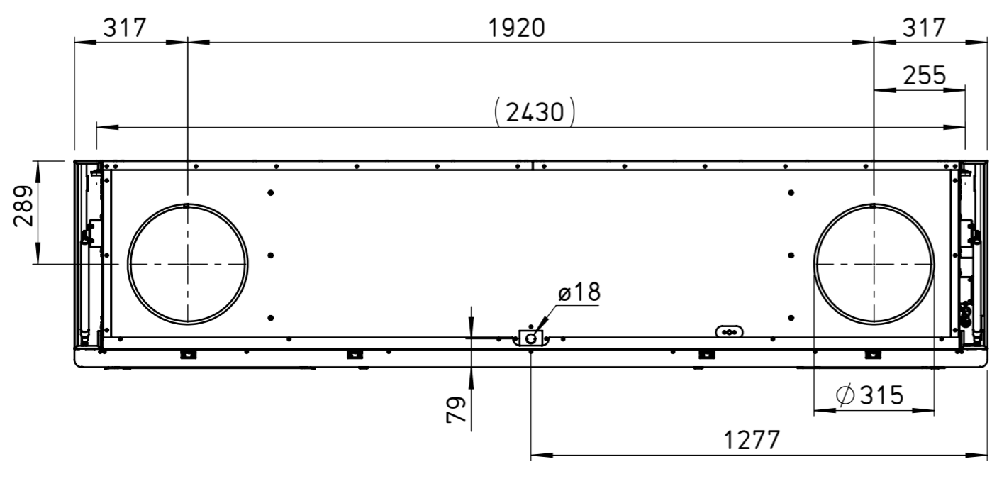
Ansicht mit Kondensatanschluss unten
