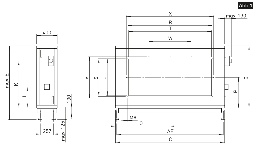
Abmessungen externe elektrische Nachheizung AIR1-ENH RH:
