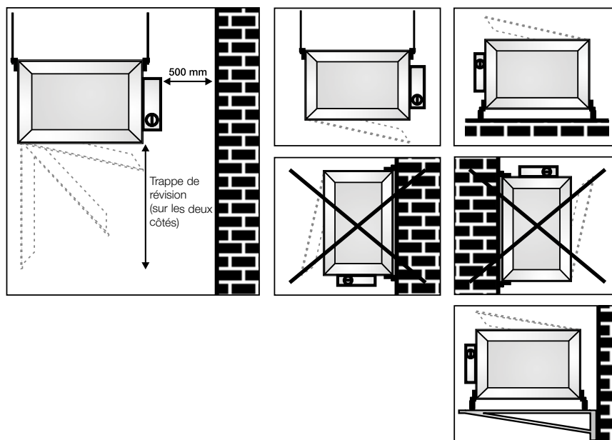
Positions de montage (aperçu côté soufflage)
