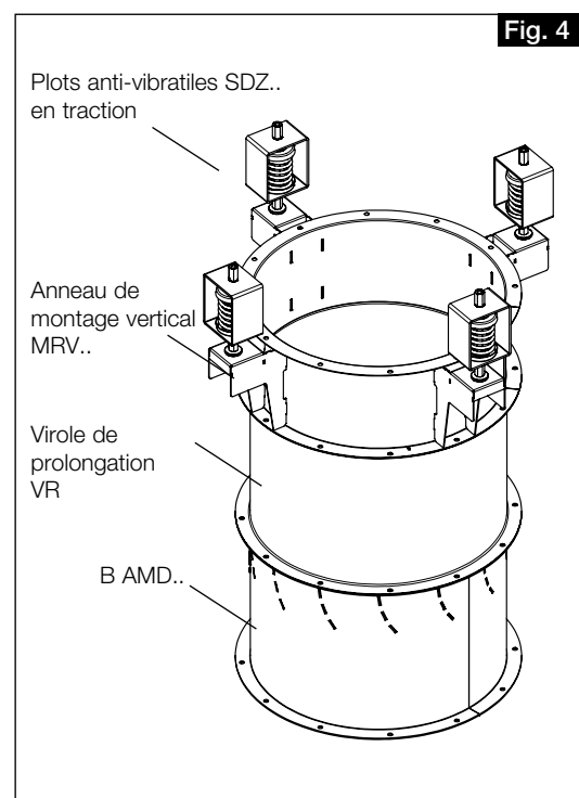
Exemples de montage – Vertical F300/400 : Ventilateur de désenfumage B AMD.. avec accessoires
