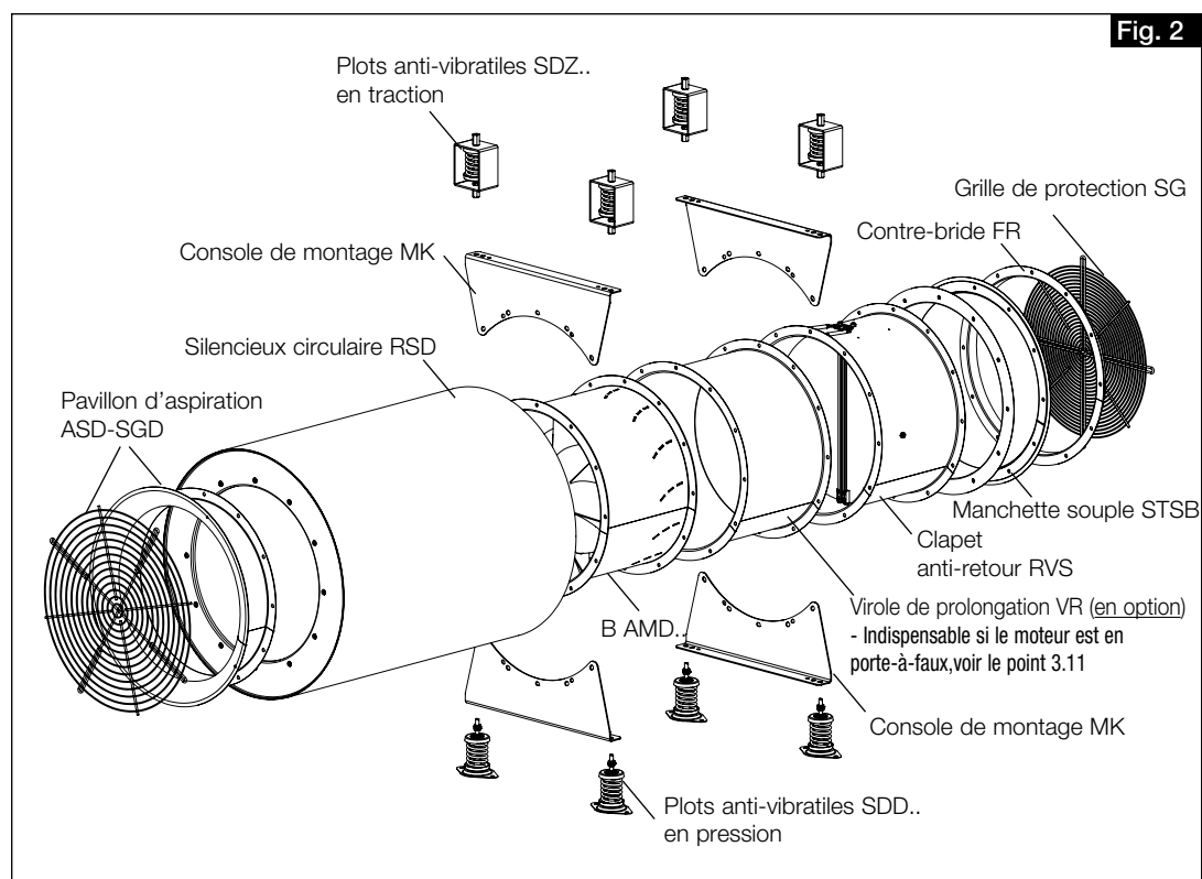
Vue d'ensemble : Ventilateur de désenfumage B AMD avec accessoires (horizontal)
