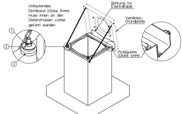
Abb. 4: Sockelschalldämpfer SSD ohne Scharnier
