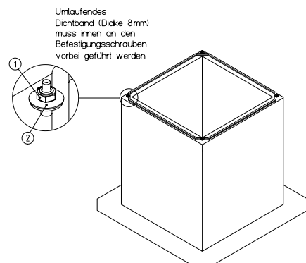
Abb. 4: Sockelschalldämpfer SSD ohne Scharnier
