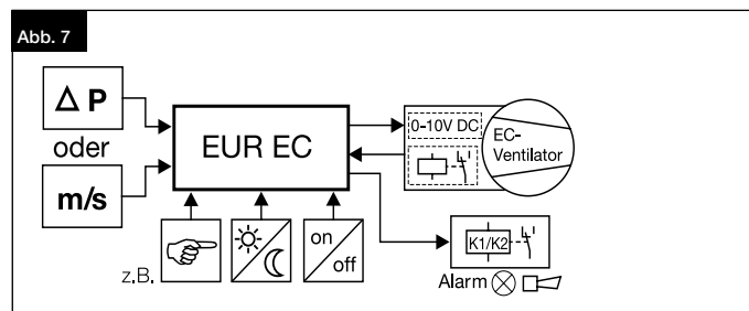
Beispiel 2: Differenzdruckregelung und Luftgeschwindigkeitsregelung
