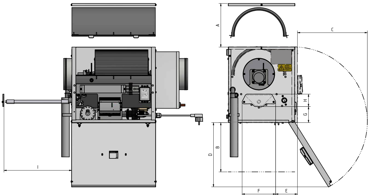
Wartungsabstände KWL HBX 250:
