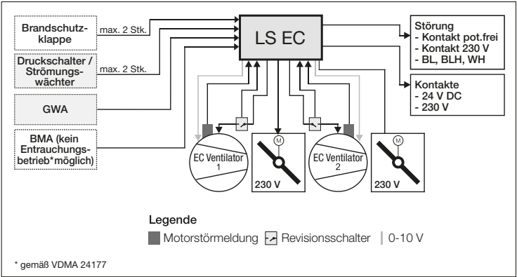
Systemskizze LS EC
