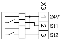
CO 2 Commande de porte ou contact GTB
