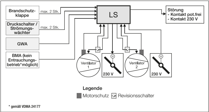
Systemskizze LS
