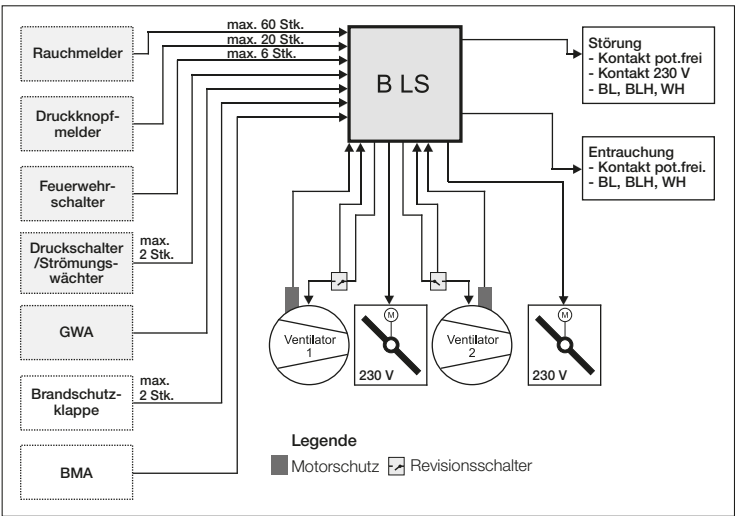
Systemskizze B LS
