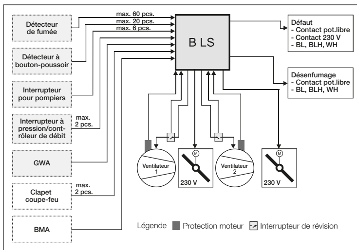
Schéma du modèle B LS avec fonction de désenfumage
