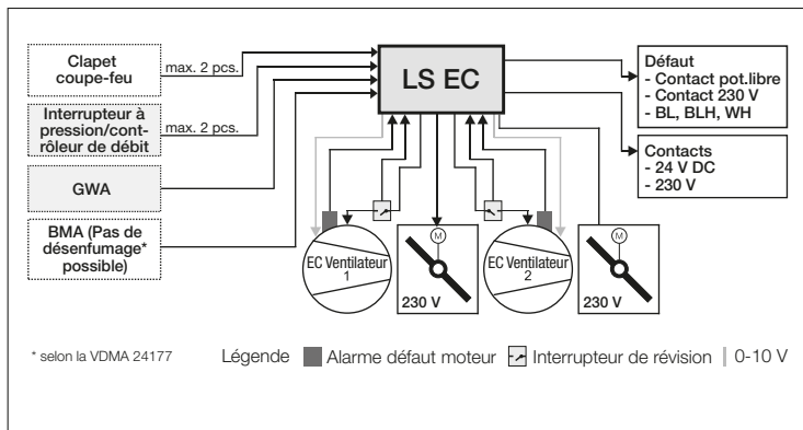
Schéma du modèle LS EC
