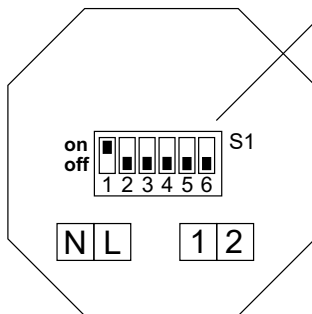
Einstellung der DIP-Schalter
